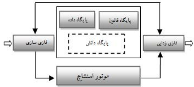
شکل ۴: شمای کلی و مراحل اصلی در یک سیستم استنتاج فازی
