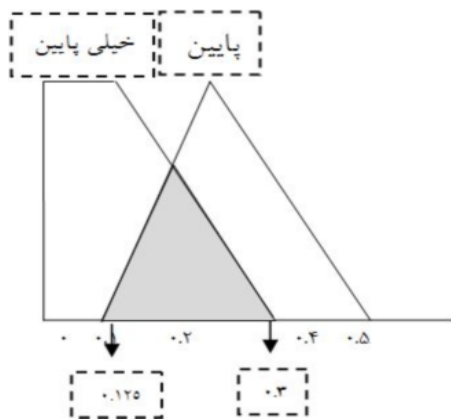
شکل ۷: نمایش گرافیکی نافازی سازی به روش مرکز ثقل منبع: نویسندگان، ۱۳۹۳
