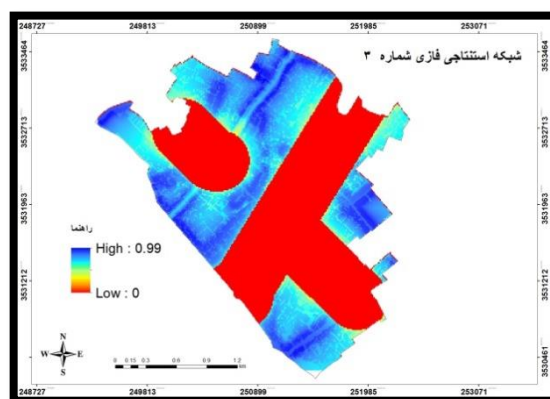
شکل ۱۴. نقشه استنتاج فازی با عملگر گاما ۸۵٪
