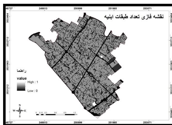
شکل ۸. نقشه لایه تعداد طبقات فازی شده
