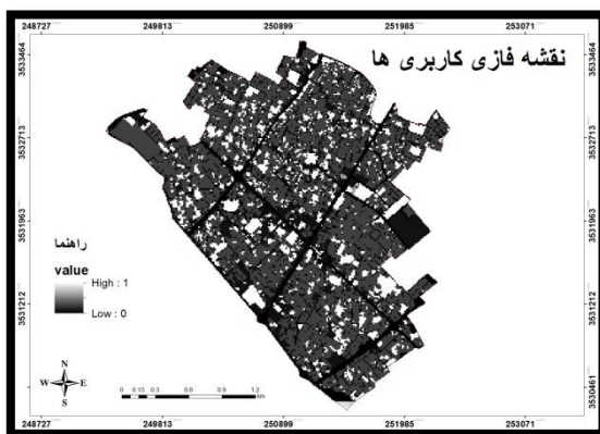
شکل ۷. نقشه لایه کاربری‌های فازی شده
