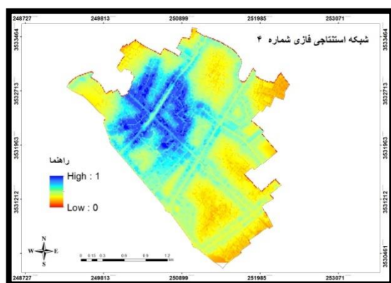
شکل ۱۵. نقشه استنتاج فازی با عملگر گاما ۹۵٪
