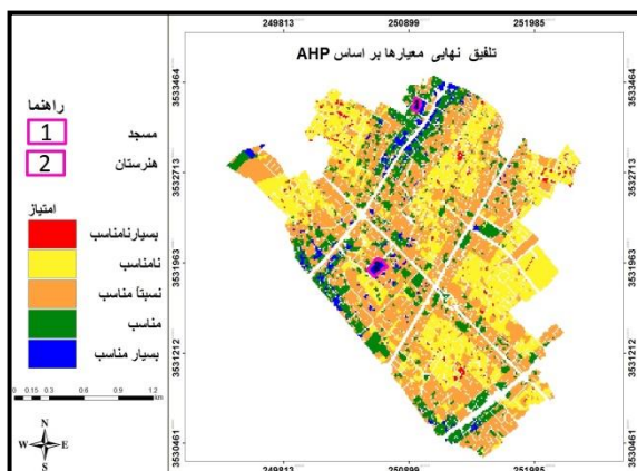
شکل ۳. نقشه گزینۀ‌های مناسب براساس مدل AHP
