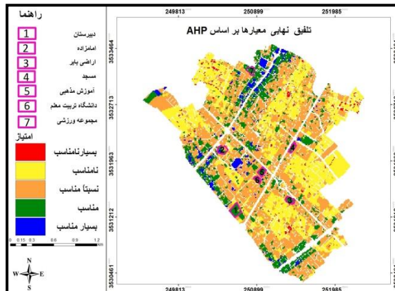
شکل ۴. نقشه گزینۀ‌های بسیار مناسب براساس مدل AHP
