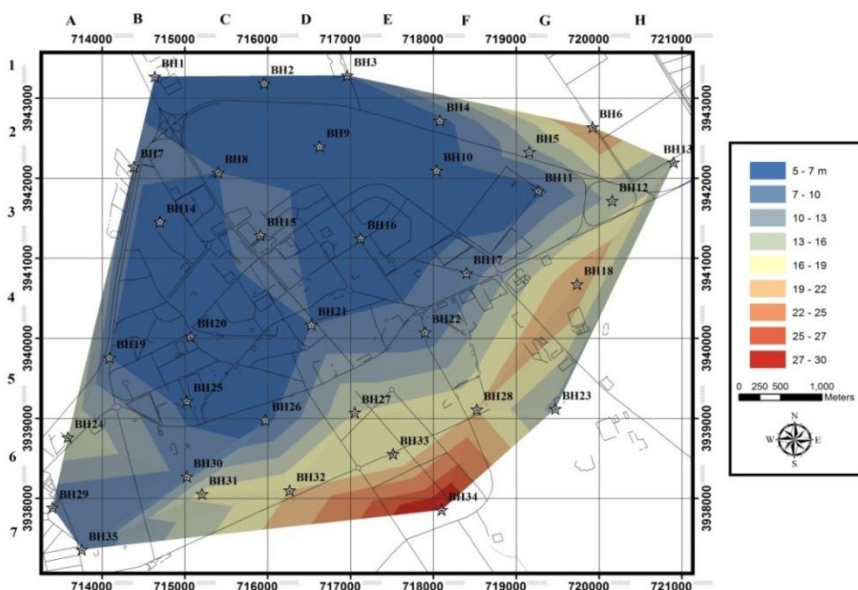
شکل ۴. ژرفای سنگ‌بستر لرزه‌ای معادل سرعت موج برشی ۷۵۰ متر بر ثانیه به روش TIN (منبع: نویسندگان، ۱۳۹۵)
