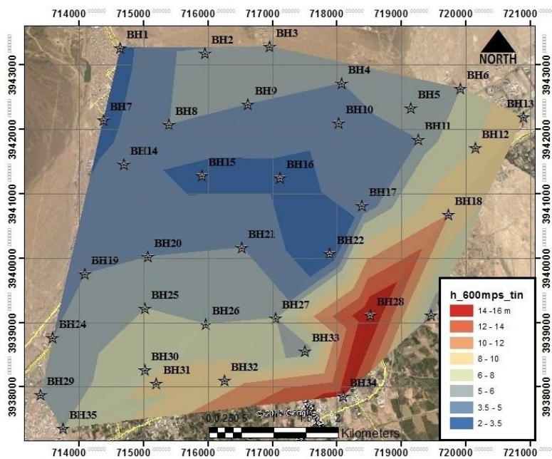
شکل ۲. ژرفای سنگ‌بستر لرزه‌ای معادل سرعت موج برشی 600 متر بر ثانیه به روش TIN
