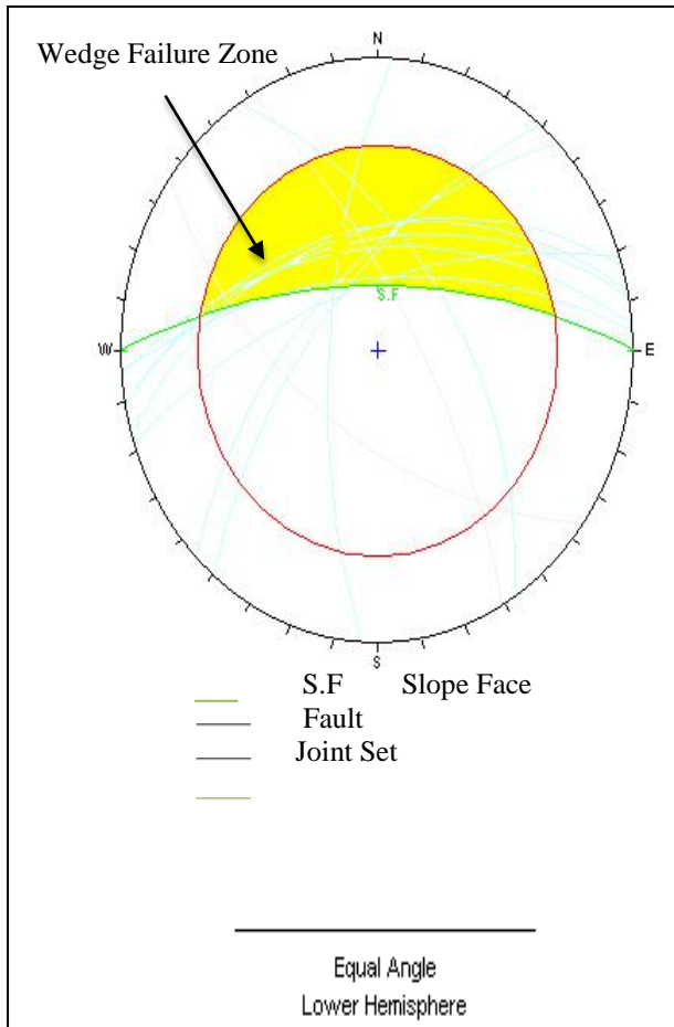
شکل ۱۷. محدوده گسیختگی گوه‌ای تکیه‌گاه چپ ( \alpha = 65^\circ ). (منبع: نگارندگان، ۱۳۹۹)
