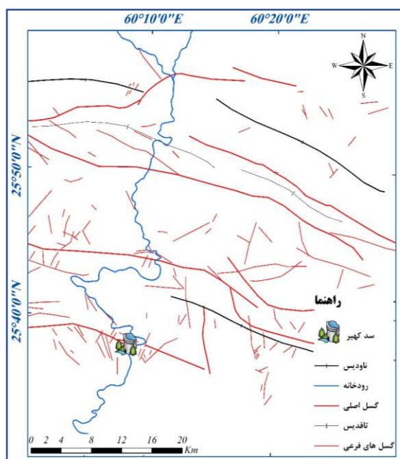
شکل ۳. نقشه ساختاری منطقه به همراه موقعیت محور سد کهریز (منبع: نگارندگان، ۱۳۹۹)
